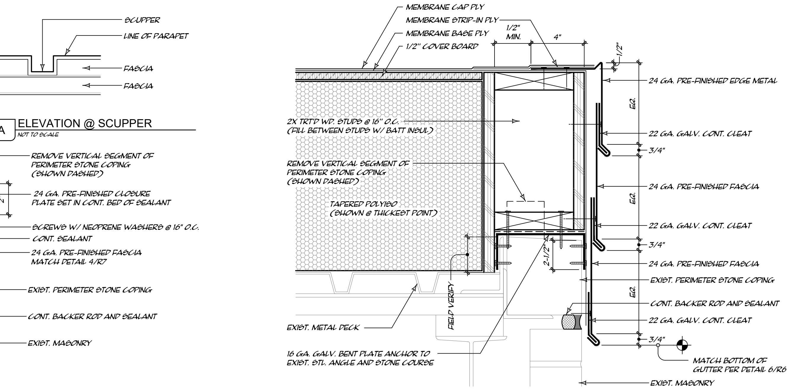
SECTION @ ROOF EDGE
